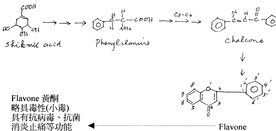
圖一 Flavone 黃酮之生合成 Biosynthesis 路徑
